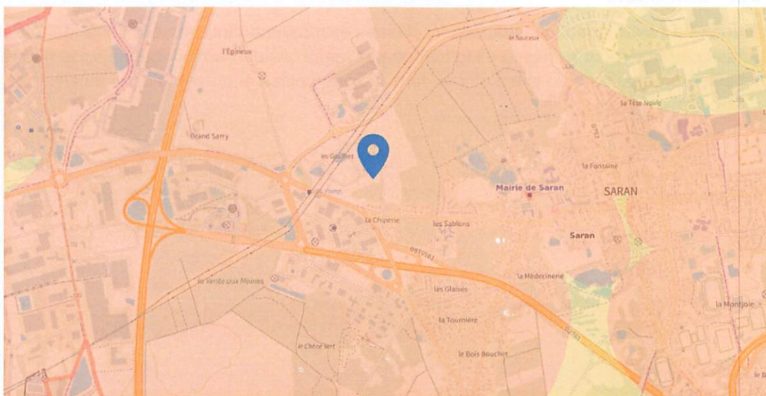
Figure 11 : Extrait de la carte "argiles" du BRGM
