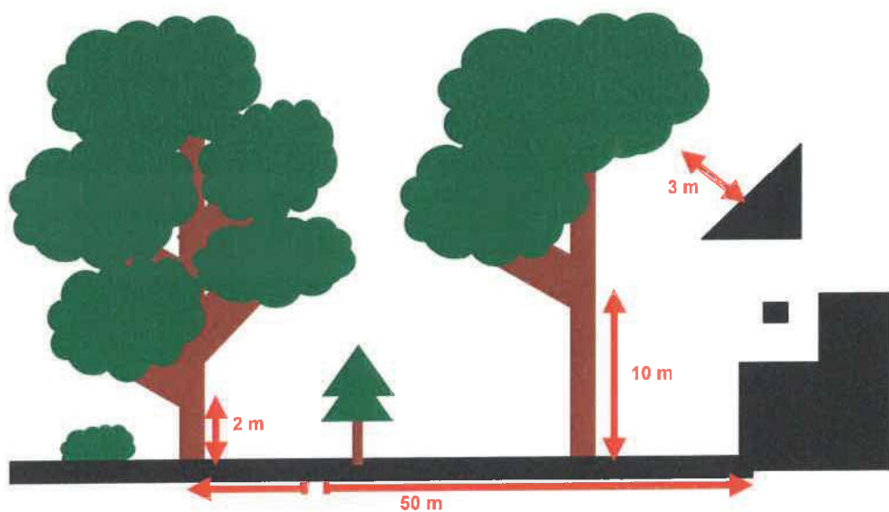
Schéma n° 3 des modalités d'application du débroussaillage pour les propriétaires de constructions : après débroussaillage .
