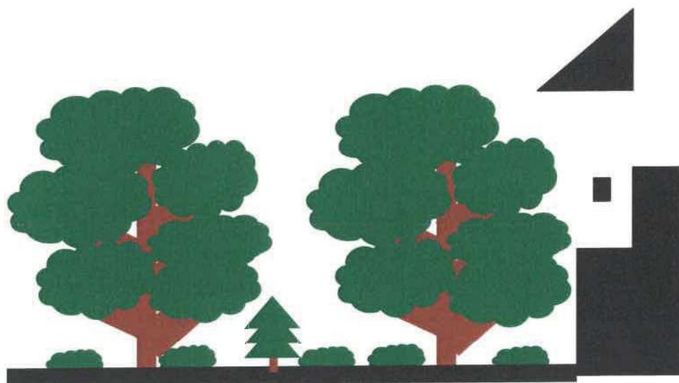
Schéma n° 2 des modalités d'application du débroussaillage pour les propriétaires de constructions : avant débroussaillage .
