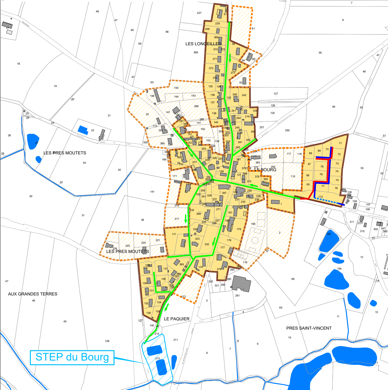
Extrait secteur assainissement collectif - Le Bourg Echelle 1/5000
