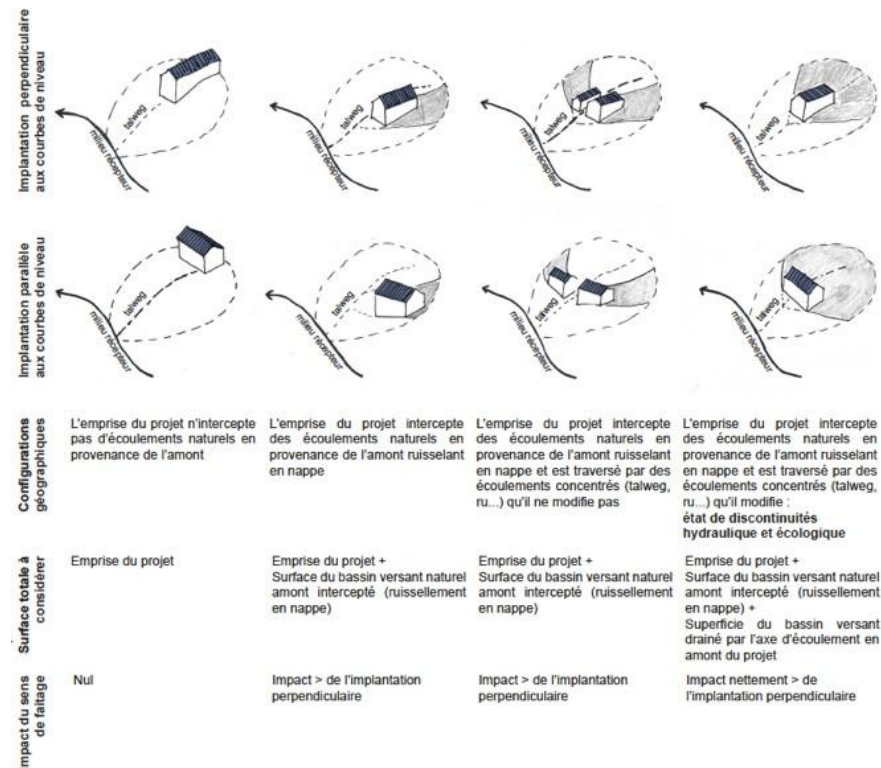
Figure 13 : Impact d'une construction sur le cycle de l'eau à l'échelle du bassin versant
