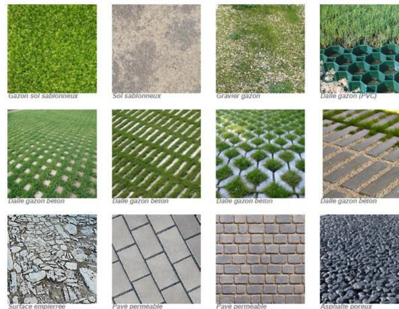
Figure 16 : Différents matériaux de revêtement des sols par ordre de perméabilité décroissante
