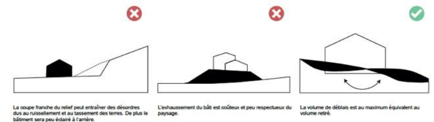
Figure 5 : Adapter la maison au terrain et non l'inverse : éviter des opérations de terrassement lourdes, privilégier une équivalence déblais/remblais
