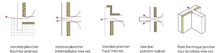
Figure 24 : Ponts thermiques les plus courants
