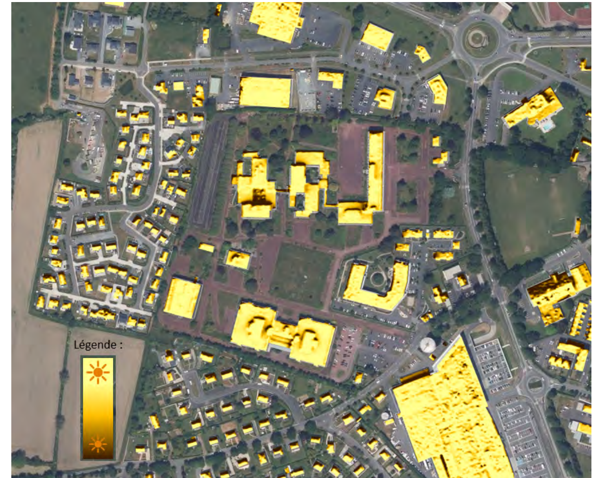
Figure 38. Potentiel solaire sur les toitures existantes sur site - Atlas solaire du Calvados
