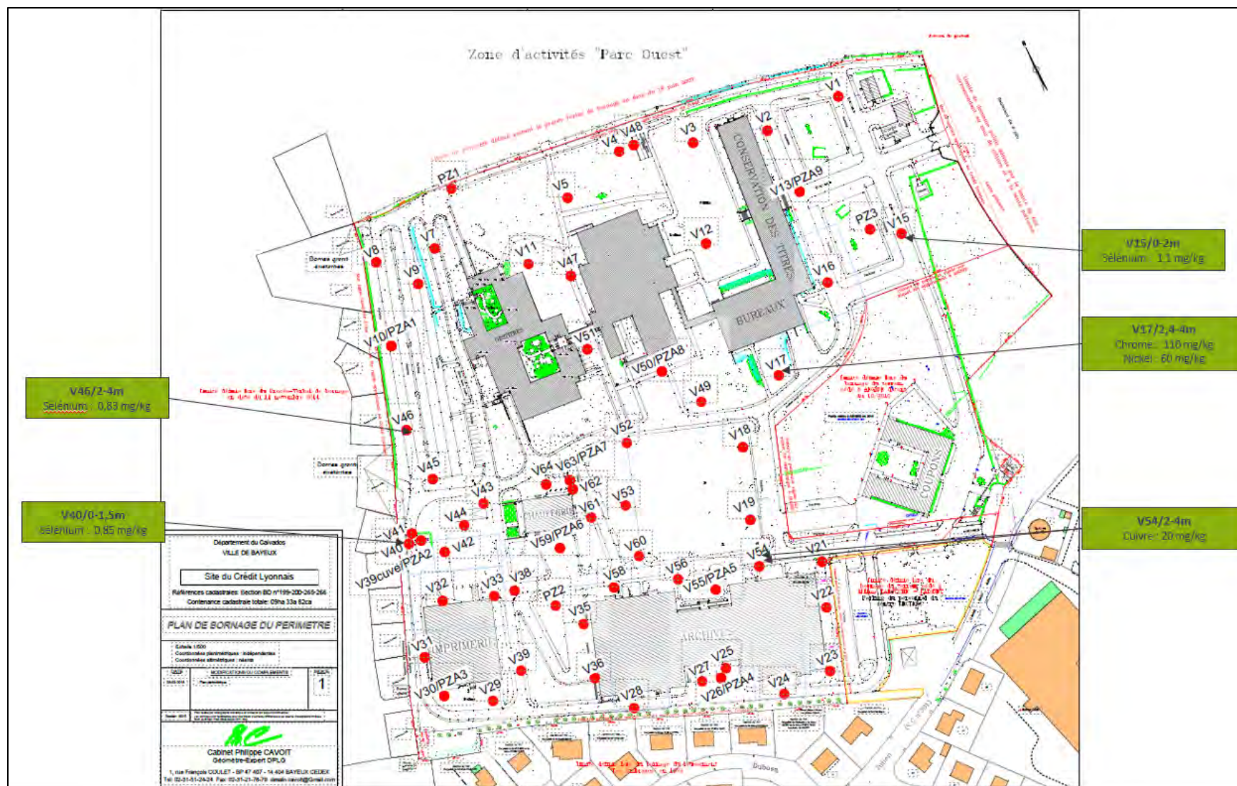
Figure 11 : Dépassement en métaux sur brut entre 0 et 4 m sur l'existant
