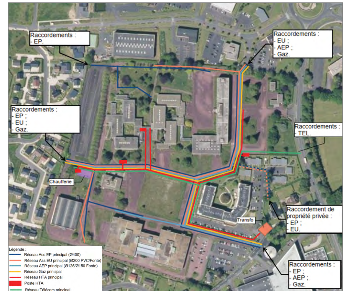
Figure 36. Réseaux sur l'ancien site du Crédit Lyonnais / La reconversion du site LCL – étude d'urbanisme pré-opérationnelle 2022
