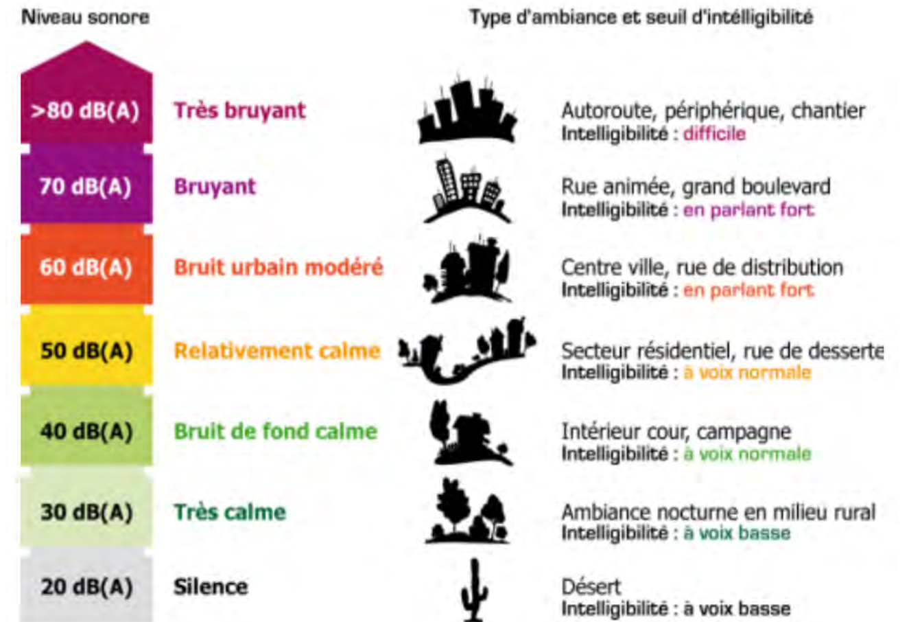
Figure 24. Echelle du bruit dans l'environnement
