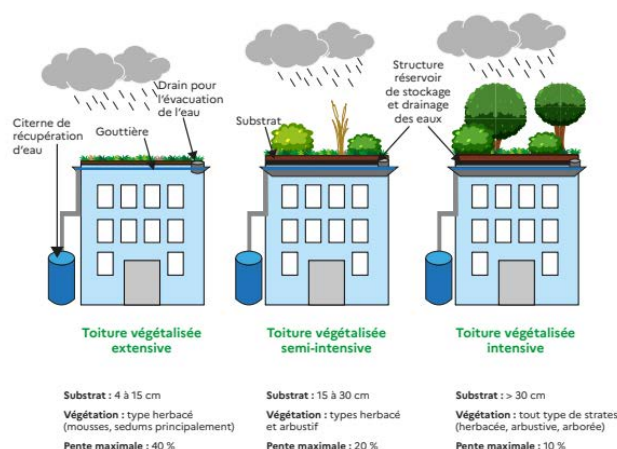
Schéma simplifié des trois types de toiture végétalisée
