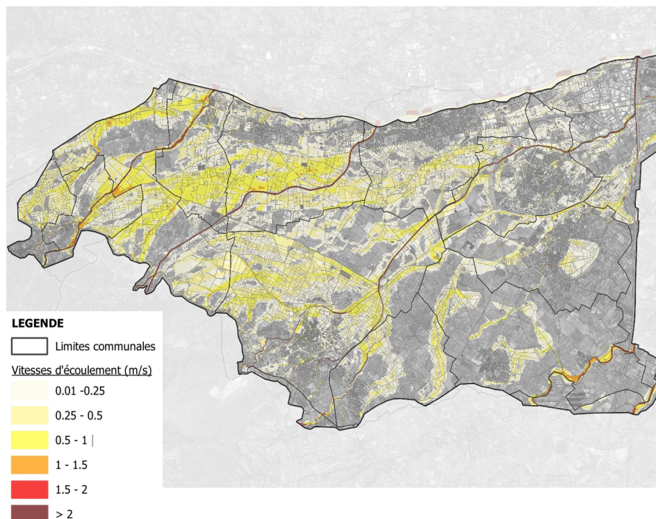
Illustration 33 : Cartographie des vitesses d'écoulement de l'eau pour la crue de référence
