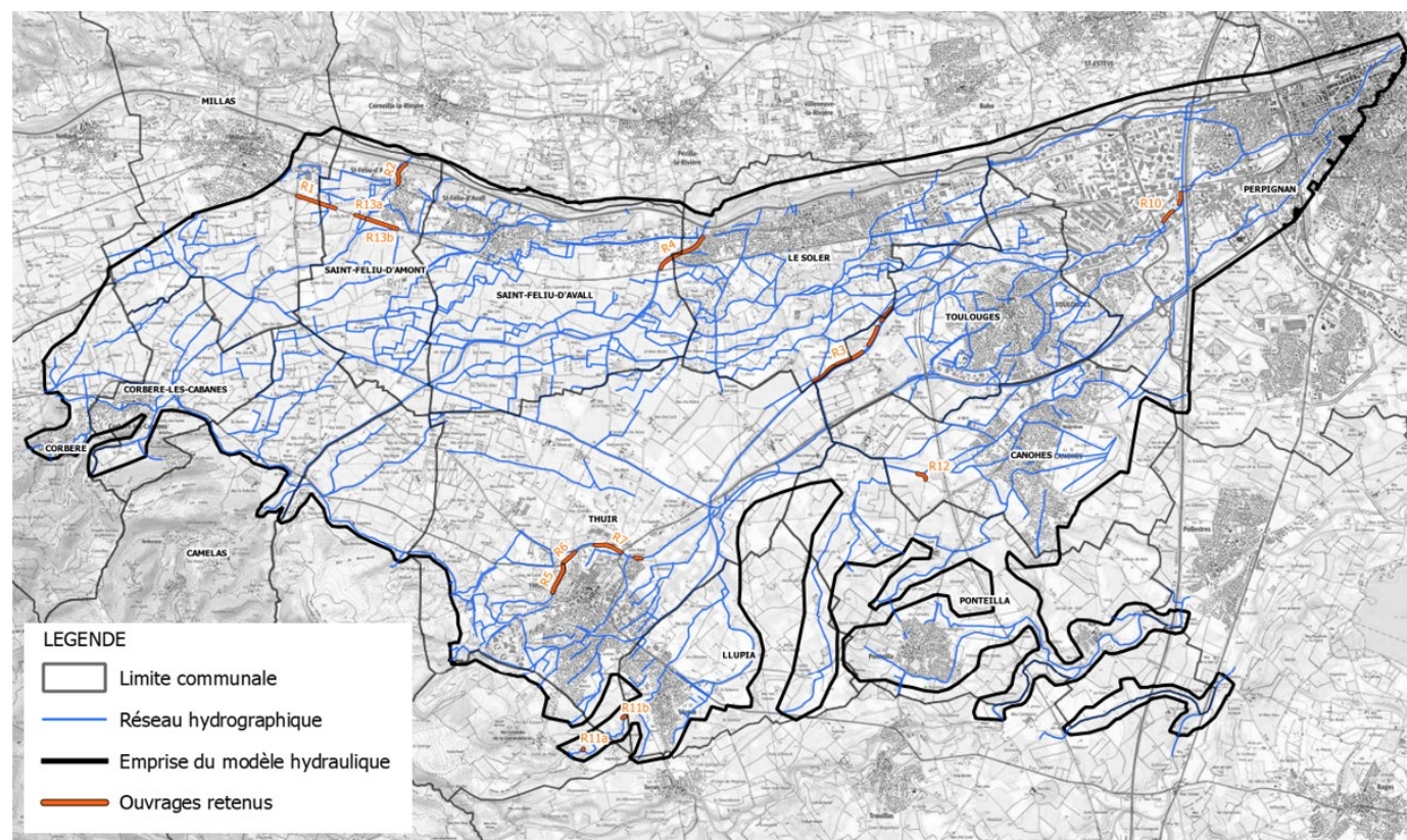
Illustration 31 : Ouvrages en remblai retenus pour l'étude des scénarii d'effacement et de rupture
