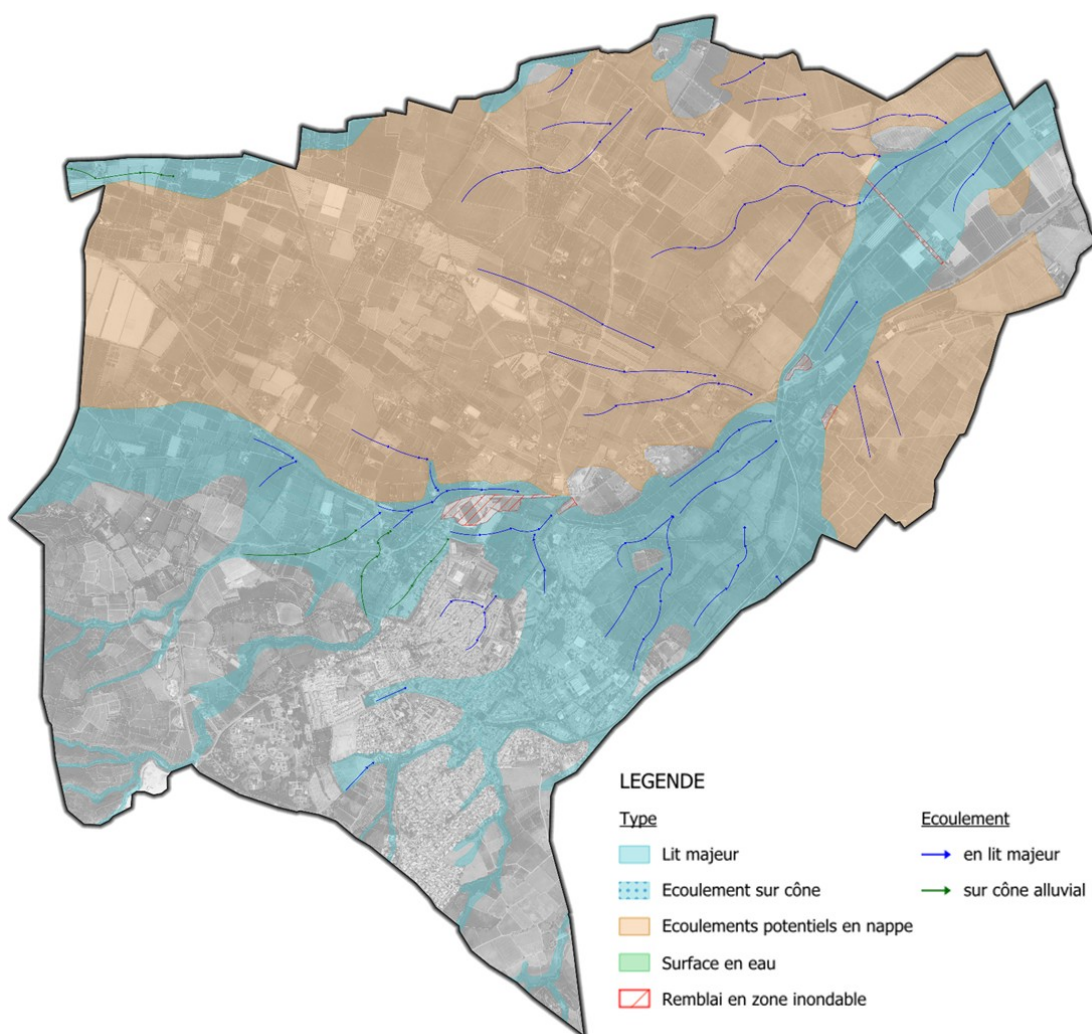
Illustration 26 : Cartographie de l'aléa hydrogéomorphologique
