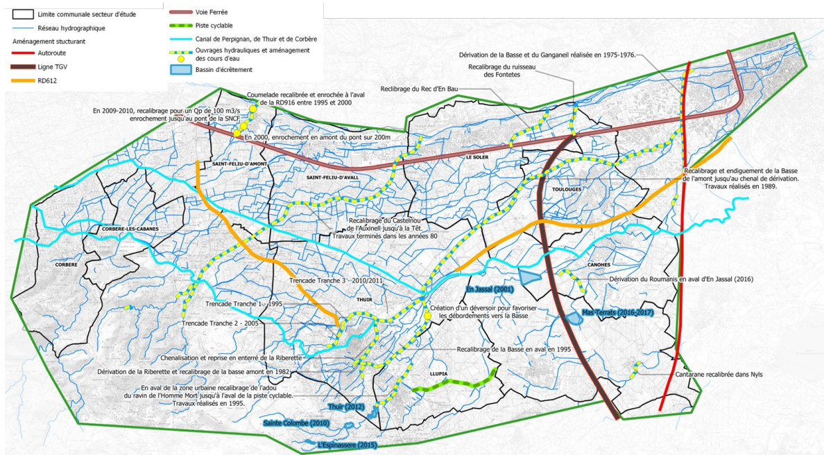
Illustration 16 : Aménagements structurants à l'échelle du bassin versant
