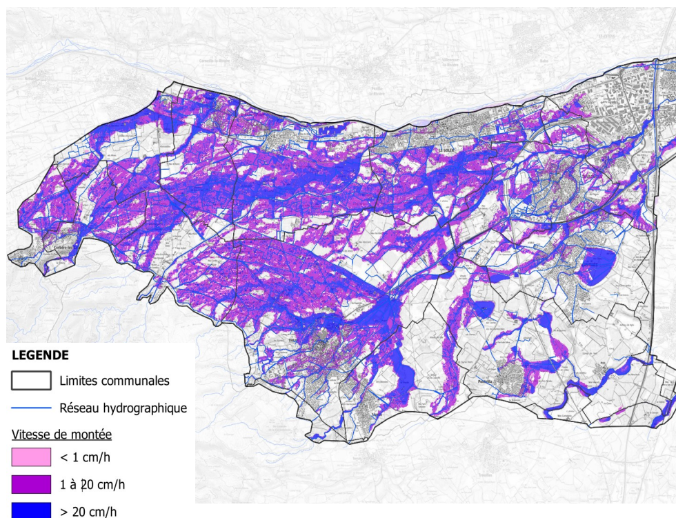
Illustration 34 : Cartographie des vitesses de montée de l'eau pour la crue de référence
