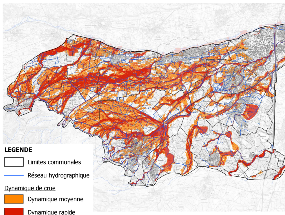
Illustration 35 : Cartographie de la dynamique de crue
