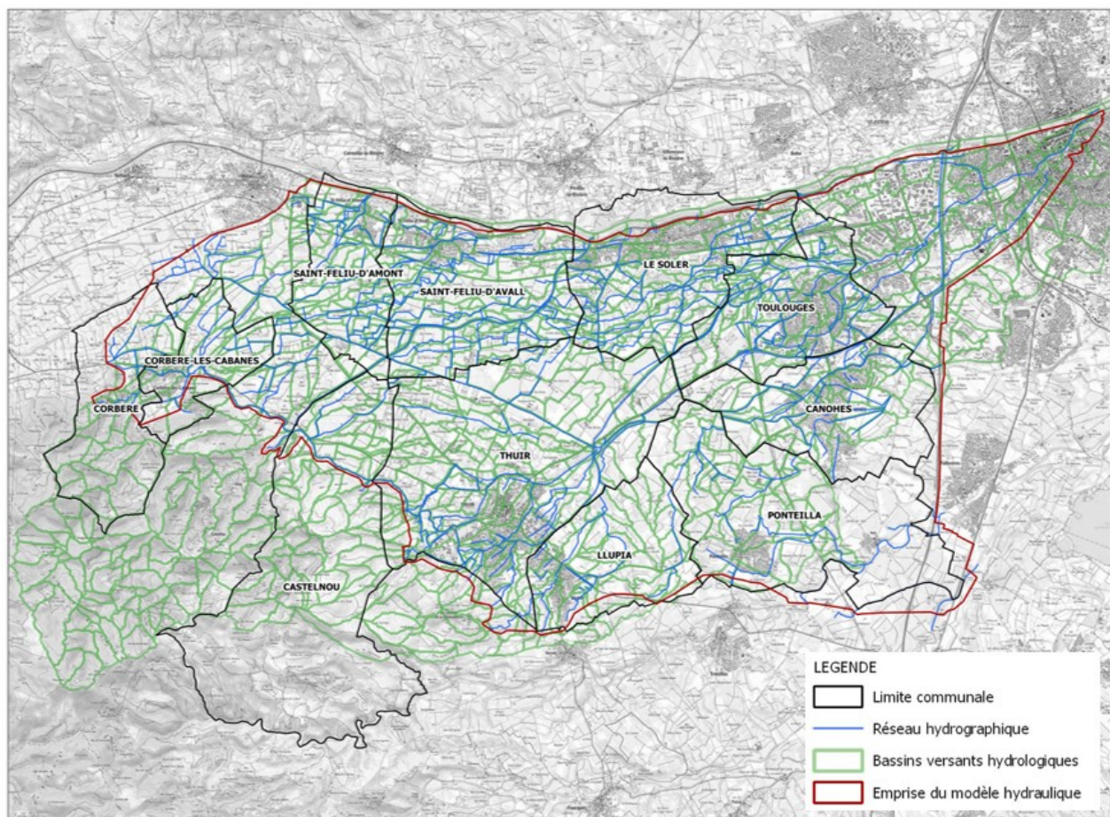
Illustration 29 : Bassins versants hydrologiques
