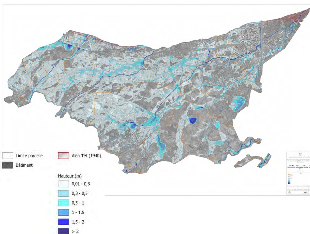
Illustration 32 : Cartographie des hauteurs d'eau pour la crue de référence
