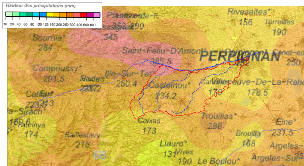
Illustration 25 : Répartition spatiale de la pluie du 29 novembre au premier décembre 2014 (source : Météo France, cumul sur 2 jours).
