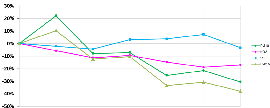
Evolution des concentrations de fond des polluants en % par rapport à 2010
