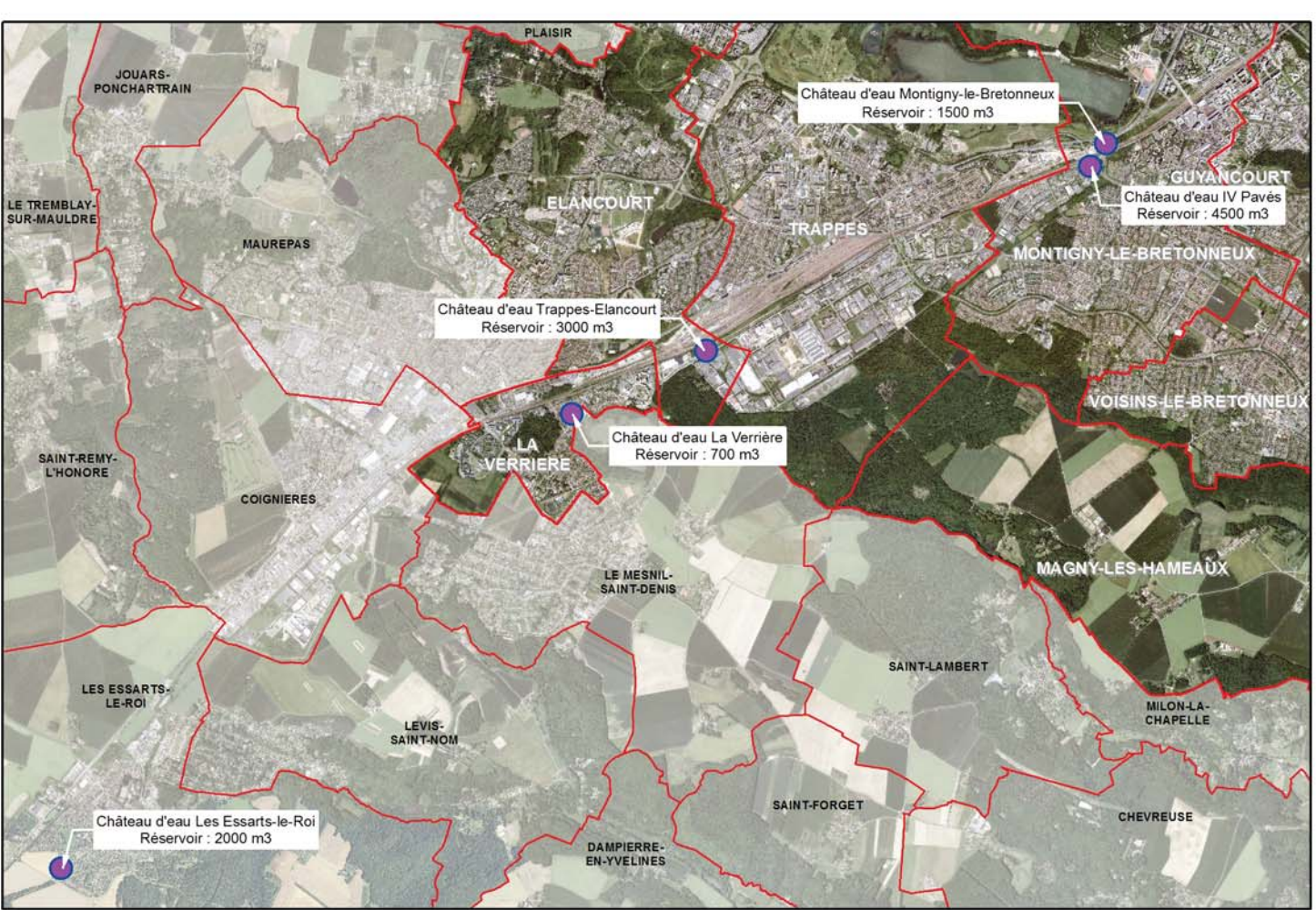
Plan de localisation des lieux de stockage d'eau potable de Saint-Quentin-en-Yvelines
