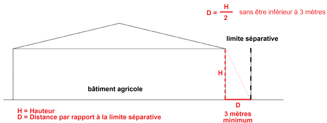
ILLUSTRATION A-3 : IMPLANTATION DES BÂTIMENTS AGRICOLES PAR RAPPORT AUX LIMITES SÉPARATIVES
