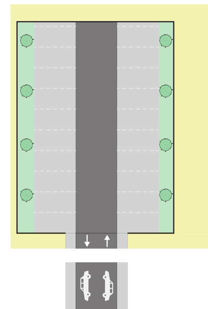
EXEMPLE DE TRANSFORMATION D'UNE AIRE DE RETOURNEMENT EN ESPACE DE STATIONNEMENT
