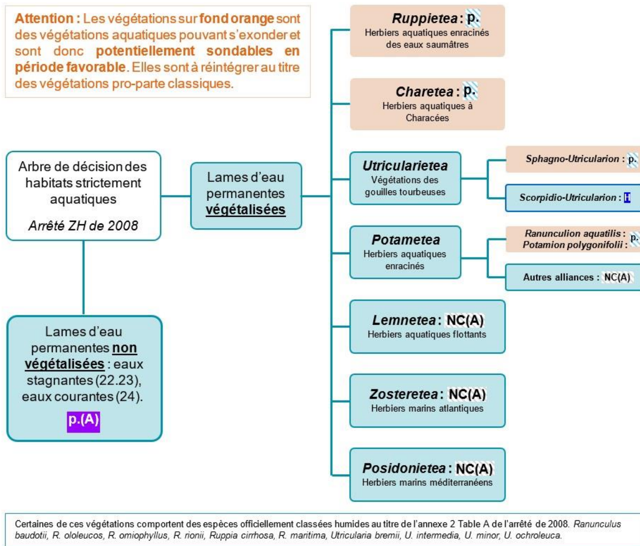
Figure 3 : Arbre de décision des habitats strictement aquatiques (© BIOTOPE)
