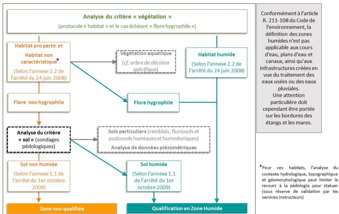
Figure 2 : Schématisation de la méthodologie de délimitation des zones humides selon la Circulaire du 18 janvier 2010, en application de l'arrêté du 24 juin 2008 (modifié par l'arrêté du 1er octobre 2009) (© BITOPE)
