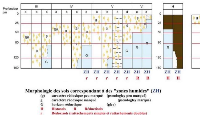
Figure 4 : Illustration des caractéristiques des sols de zones humides (GEPPA, 1981)
